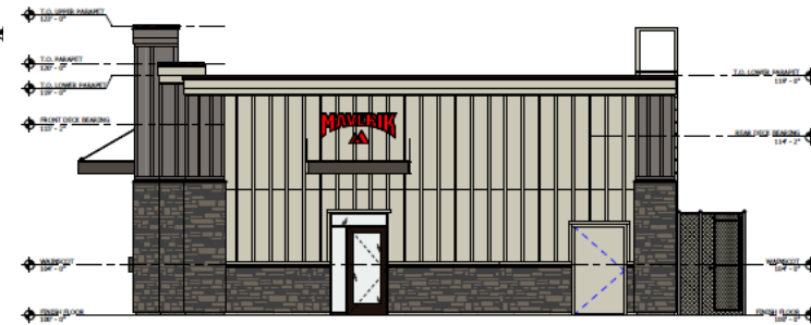
2 RIGHT ELEVATION SCALE: 1/4" = 1'-0"
