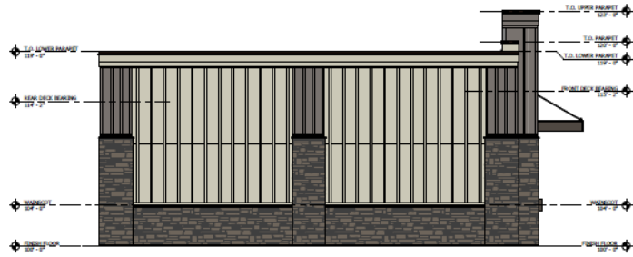
2 LEFT ELEVATION SCALE: 1/4" = 1'-0"
